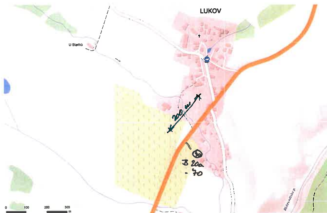
Situační plán s vyznačením navrhovaného umístění dopravního značení č. B20a-70
