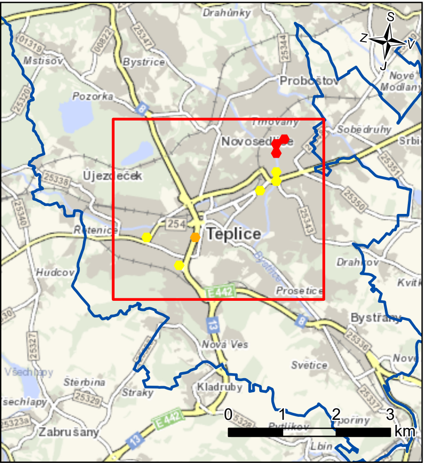
Mapa č. 2 - Vymezení kritických míst pro hluk z dopravy na řešených pozemních komunikacích
