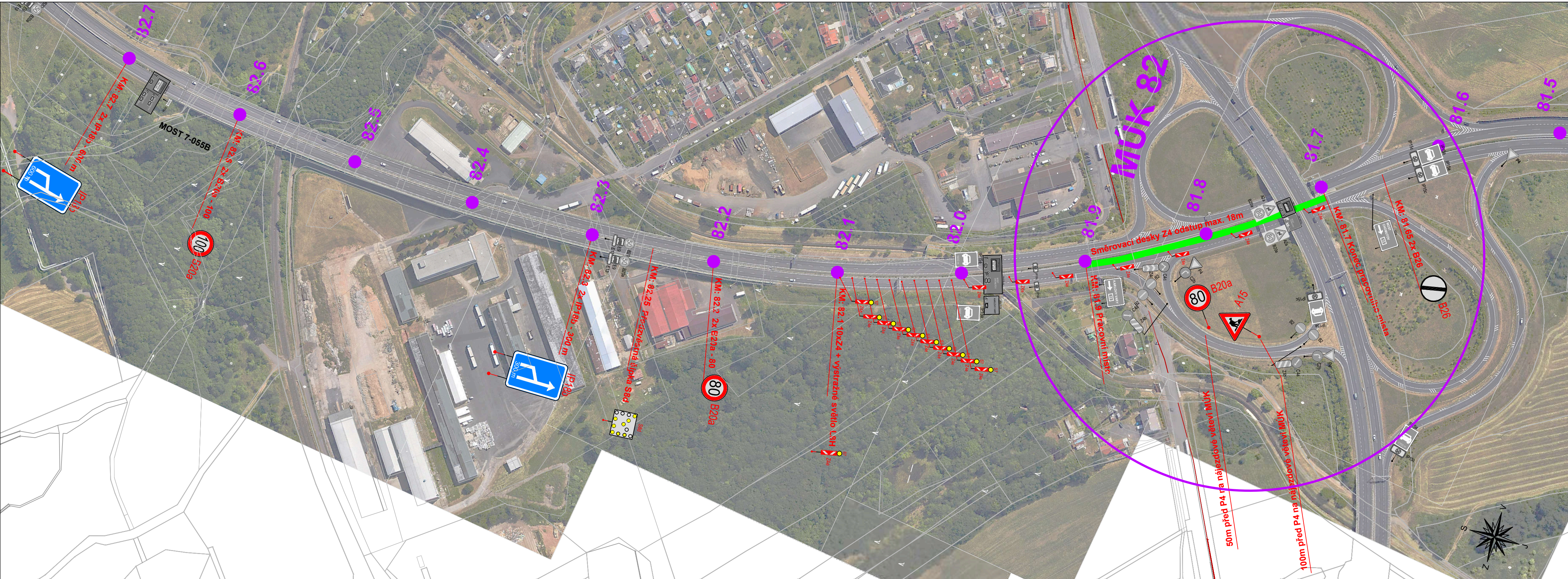
Výřez 2: Km: 84.1 - 82.6
