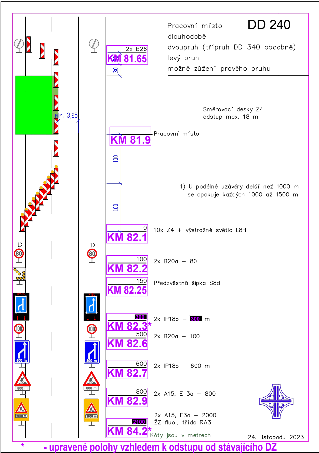
Schéma DIO včetně staničení
