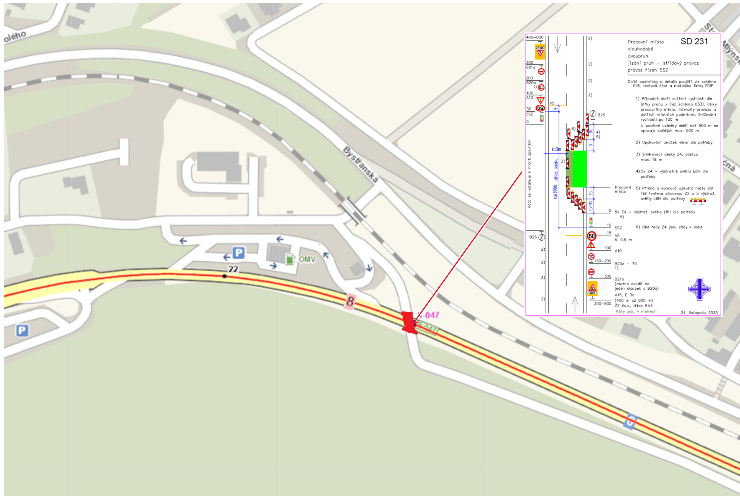
DETAIL č. 2 – částečná uzavírka – I/8 pod mostem
