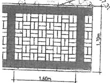
ADEČSKÉ SCHÉMA DLAŽBY CHODNIČKU
